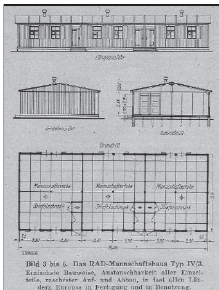
Szkic podstawowego baraku mieszkalnego typu RAD, źródło: internet
