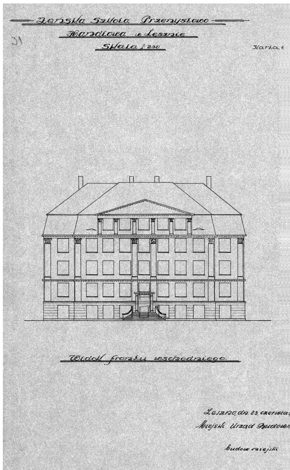
20. Projekt elewacji wschodniej niezrealizowanej Żeńskiej Szkoły Przemysłowo-Handlowej w Lesznie, 23 czerwca 1927 r.
