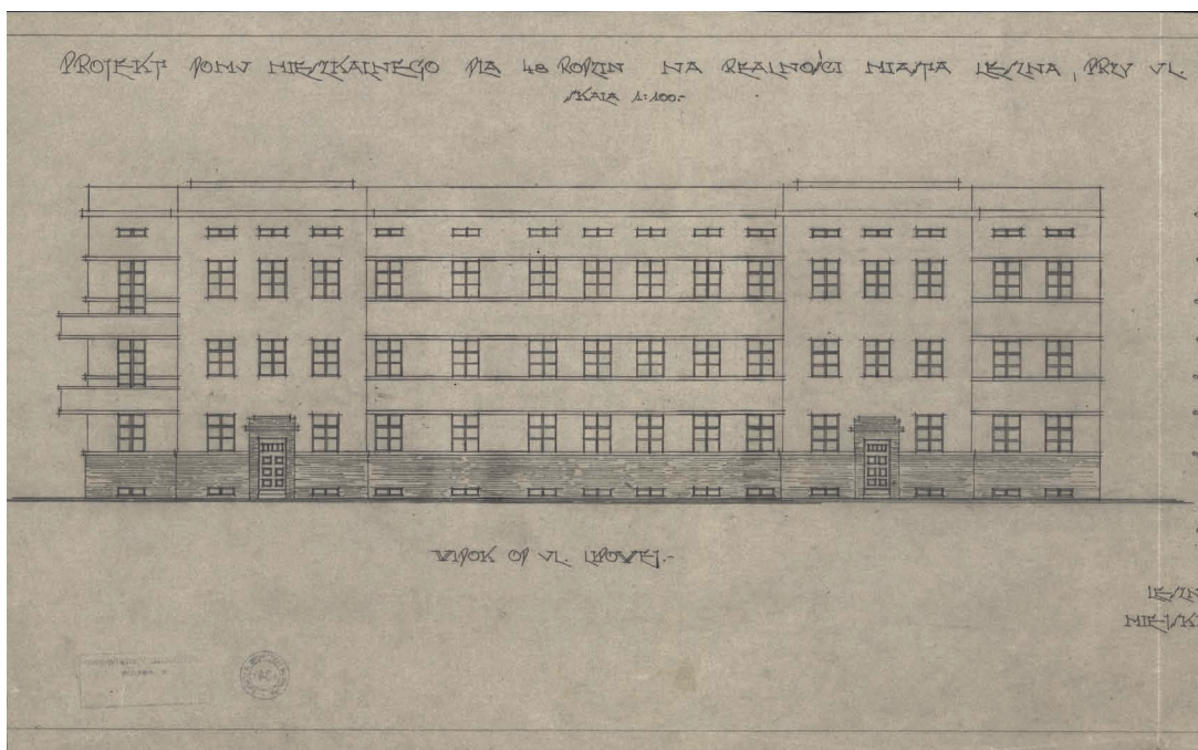
13. Projekt 48-rodzinnego domu mieszkalnego u zbiegu ob. ul. Lipowej i Strzeleckiej w Lesznie, widok od strony ul. Lipowej, 1929 r.
