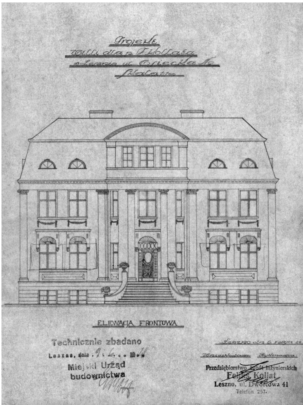
17. Projekt willi Feliksa Kollata, elewacja frontowa – fasada, 6 maja 1928 r.
