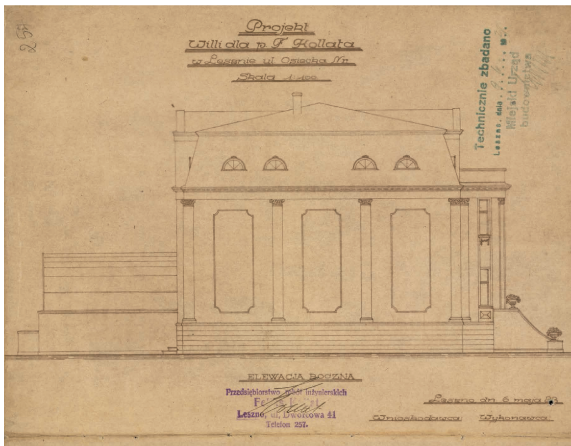
15. Projekt willi dla Feliksa Kollata, elewacja boczna, 6 maja 1928 r.
