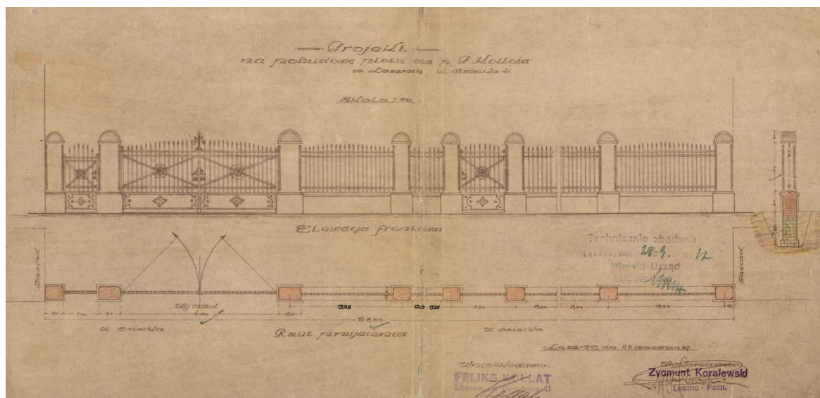
14. Projekt budowy parkanu przy willi Feliksa Kollata, widok i rzut przyziemia, 22 września 1927 r.
