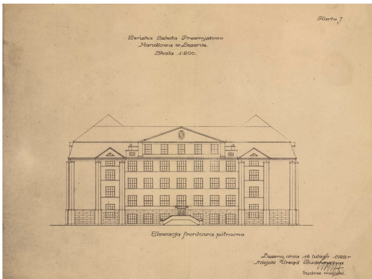
5. Wizualizacja niezrealizowanej Żeńskiej Szkoły Przemysłowo-Handlowej w Lesznie, elewacja frontowa północna, 16 lutego 1928 r.
